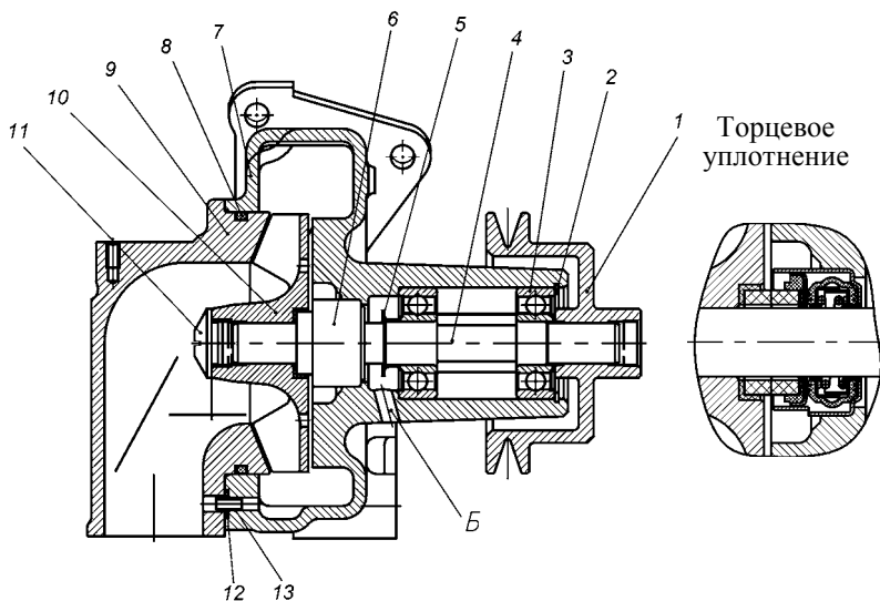
Рис. 31. Водяной насос:
