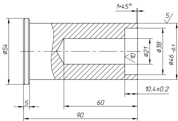
Рис. 111. Оправка
