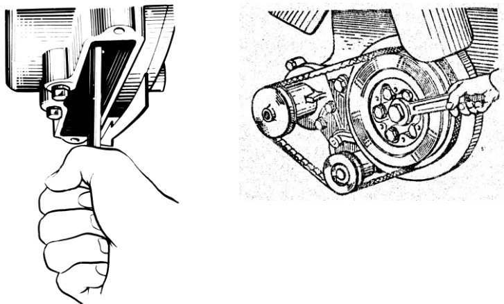
Рис. 48. Проворачивание коленчатого вала
