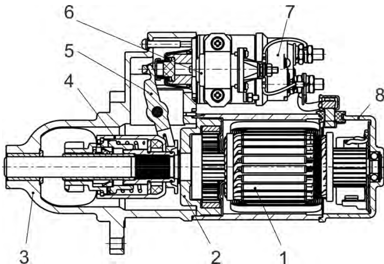
Рисунок 125 – Стартер 5432.3708-01:
