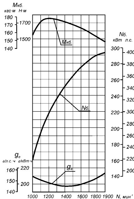
Рис. 3. Скоростная характеристика двигателей: а) ЯМЗ-7511.10; б) ЯМЗ-7512.10
