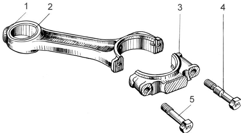
Рис. 10. Шатун:
