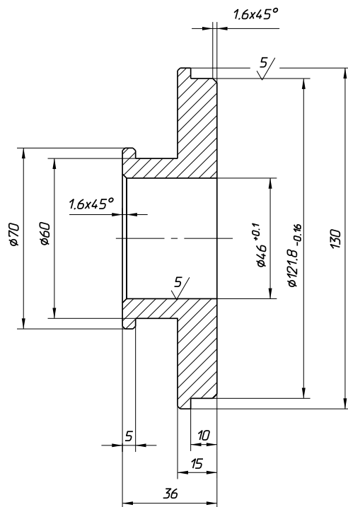
Рис. 110. Кондуктор
