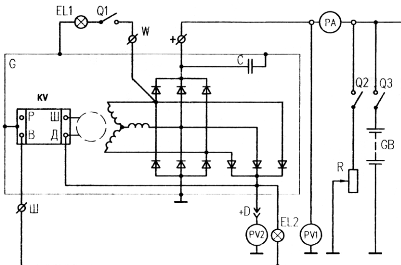
Рис. 67. Схема для проверки электрических характеристик: G—генератор; GB—аккумуляторная батарея; C—конденсатор 2,2 мкф \pm 20%; R—сопротивление нагрузки; PV1, PV2—вольтметры; PA— амперметр; KV—регулятор напряжения; Q1-Q3—выключатели; EL1, EL2—контрольные лампы-2Вт, 28В; «+», «Ш», «W», «+D»—выводы генератора.
