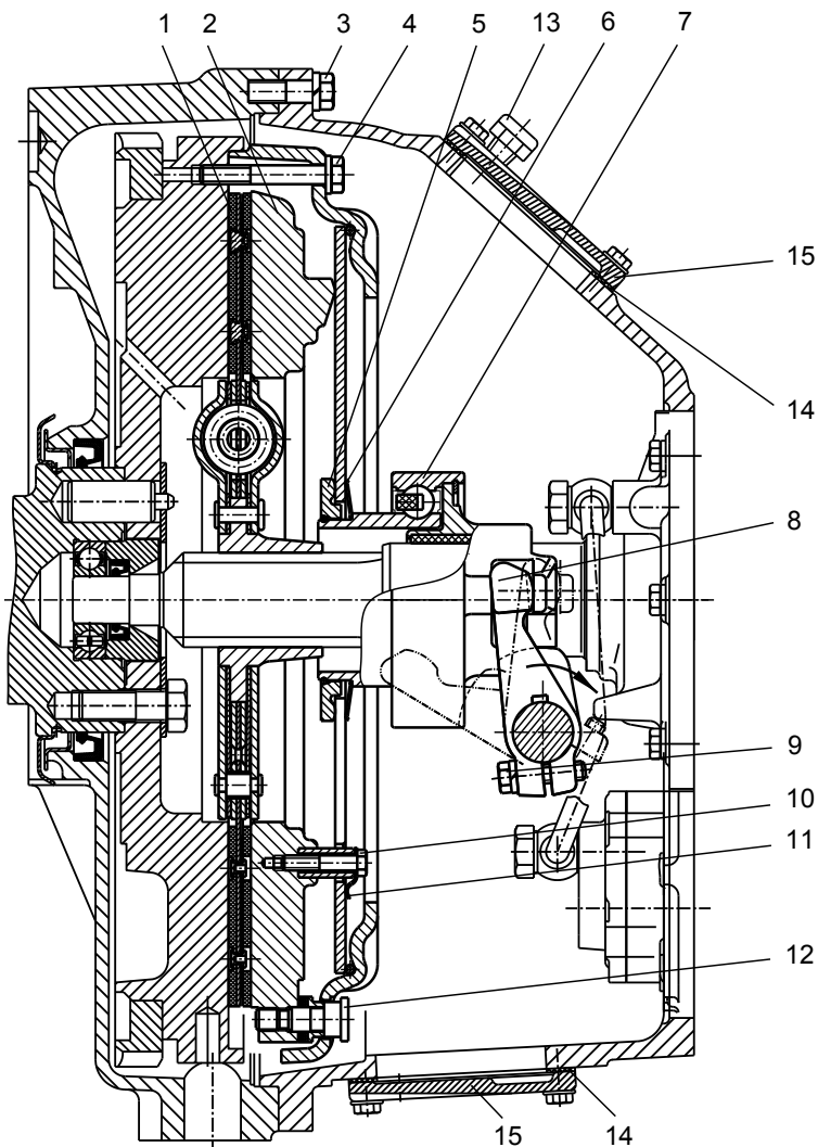
Рис. 120. Сцепление ЯМЗ-183-35:
