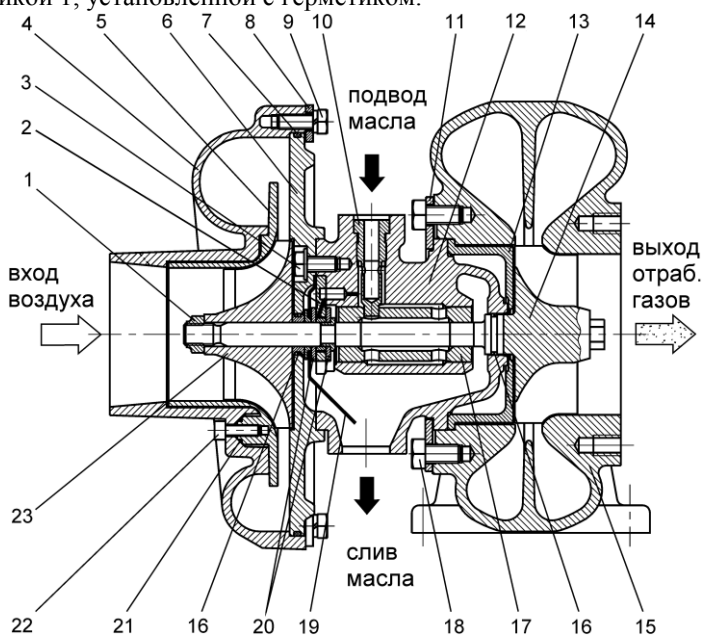
Рис. 29. Турбокомпрессор:
