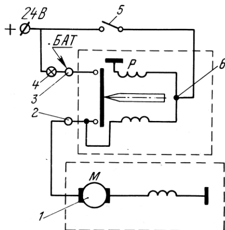
Рис. 71. Схема проверки замыкания контактов реле:
