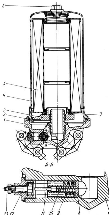
Рис. 16. Масляный фильтр:
