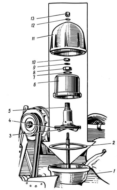
Рис. 56. Фильтр центробежной очистки масла:
