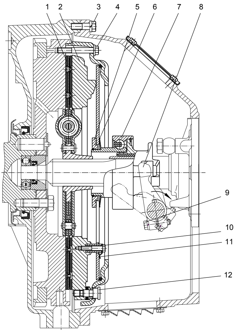
Рис. 115. Сцепление:
