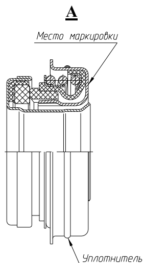
Рис.107. Водяной насос с торцовым уплотнением "KACO"
