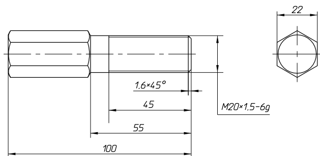
Рис. 112. Установочный винт
